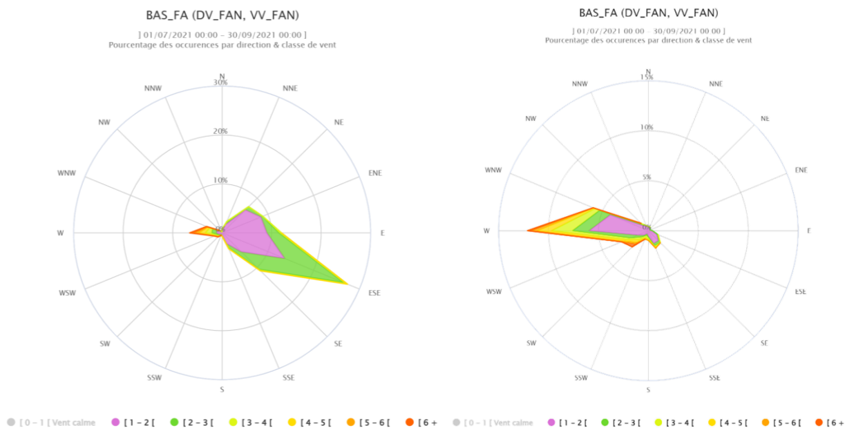
Figure 10 : Rose des vents la journée, station du Fango
