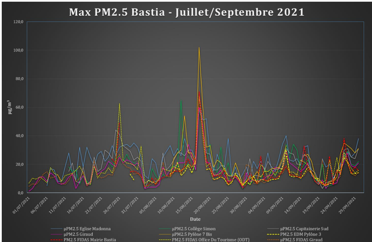
Figure 50 : Mesures Max journaliers PM 2.5 Bastia – Période Estivale 2021 – Micro-capteurs (µPM 2.5 ) et analyseurs (PM 2.5 )
