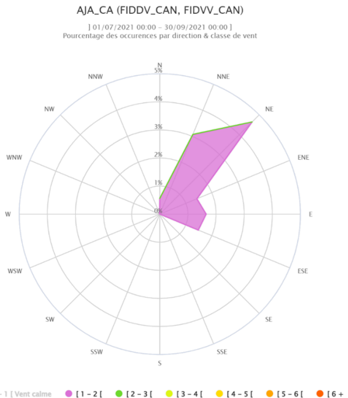
Figure 5 : Rose des vents sur Canetto - Période Estivale 2021
