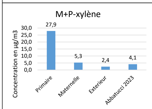
Figure 2 : Histogrammes des niveaux de concentration en BTEX à l'école de Murato
