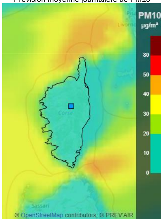
Mardi 18 janvier 2024 Prévision moyenne journalière de PM10
