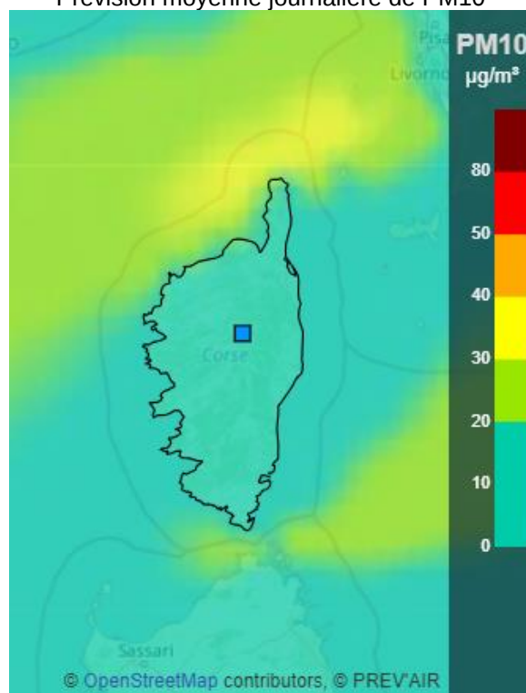
Mercredi 19 janvier 2024 Prévision moyenne journalière de PM10
